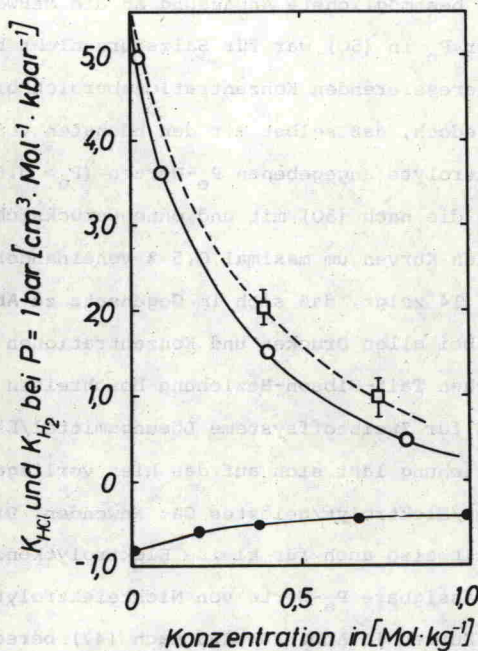
Abb. 15. Partielle molale Kompressibilität von gelöstem Wasserstoff bei Atmosphärendruck in Abhängigkeit von der HCl-Konzentration (O), bzw. von der NaCl/HCl-Konzentration ( \square ), wobei m_{HCl} \ll m_{NaCl} .
